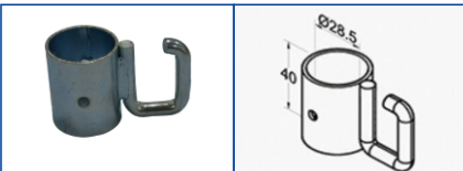
K-1012K
