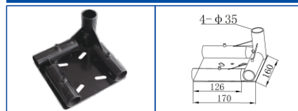
K-1003P
