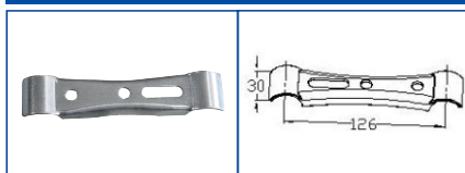
K-1002R
