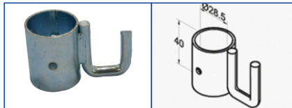
K-1012L
