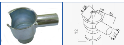
K-200 L:200/400/600MM
