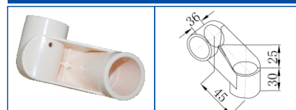
J-012
