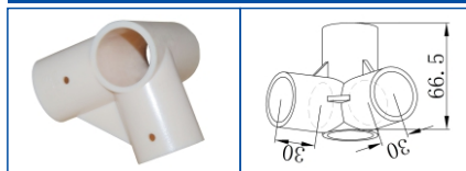
J-006
