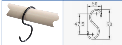
K-1012F
