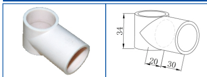
J-003A
