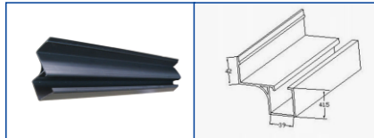
K-2080B
