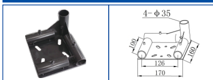
K-1003Y
