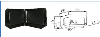
J-B3-5
