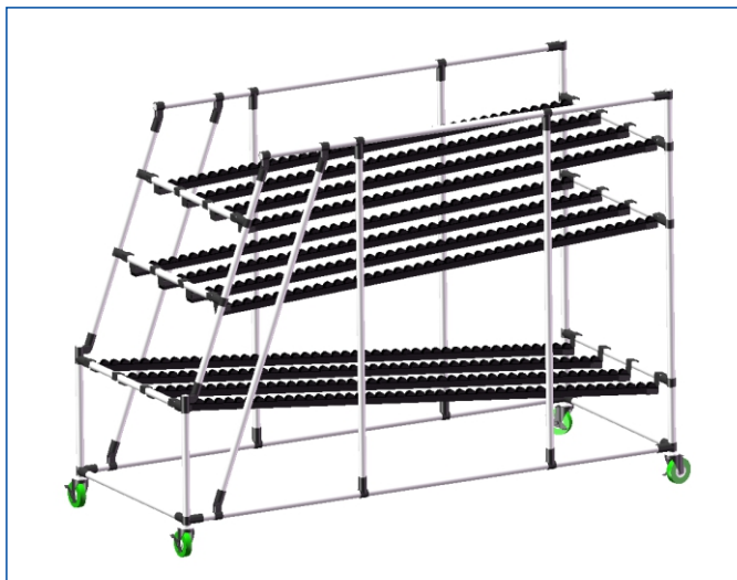
工具推车
