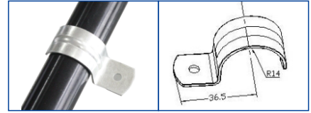
K-1009
