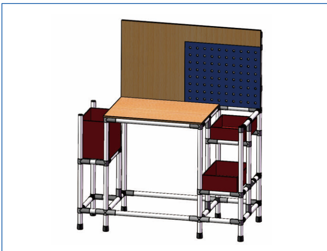
产品组装桌
